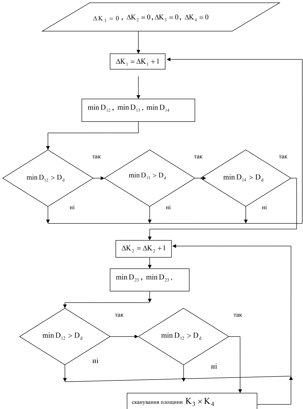
Рис. 1. Алгоритм пошуку оптимальної стратегії розходження
