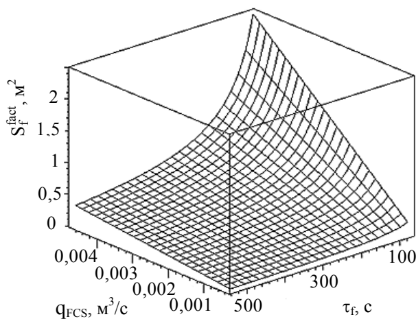
Рис. 4. Зависимость площади пожара S_f^{fact} от расхода воды из ПКК q_{FCS} и времени свободного развития пожара \tau_f , если время подачи воды \tau_{ex}=71,2 с
