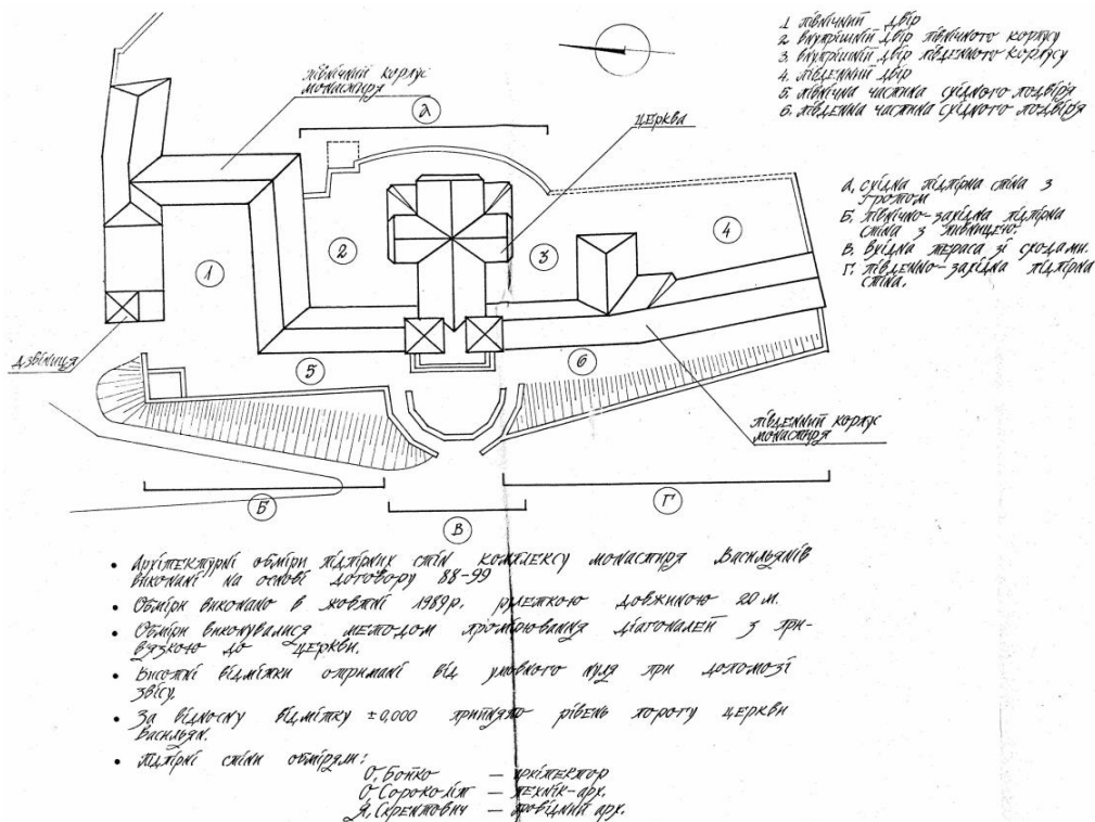
Рис.1. Схема розташування будівель монастиря (обмірні креслення). Фото із архіву Тернопільського обласного відділу в справах будівництва та архітектури
