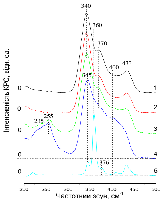
Рис.1. Нерезонансні спектри макро-Раман з Фур'є трансформацією c\text{-GeS}_2(T_x, V_y) , зняті при довжині хвилі збудження \lambda_{36.1}=1064 нм. (1.17 eВ, Nd:YAG, Bruker IFS 66/FRA 106): 1) T_1, V_1 ; 2) T_2, V_2 ; 3) T_3, V_2 ; 4) T_4, V_2 , 5) \beta\text{-GeS}_2
