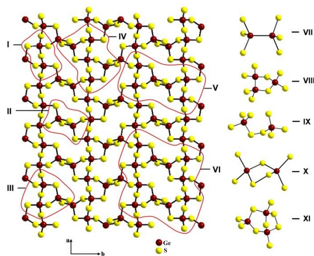
Рис.2. Зліва – моношар з кристалічної структури високотемпературної фази \beta\text{-GeS}_2 з виділеними кластерами \text{Ge}_n\text{S}_m (I–VI) та справа – “дефектні” кластери \text{Ge}_n\text{S}_m з гомеоплярними зв'язками Ge-Ge (VII–VIII) та S-S (IX–XI)
