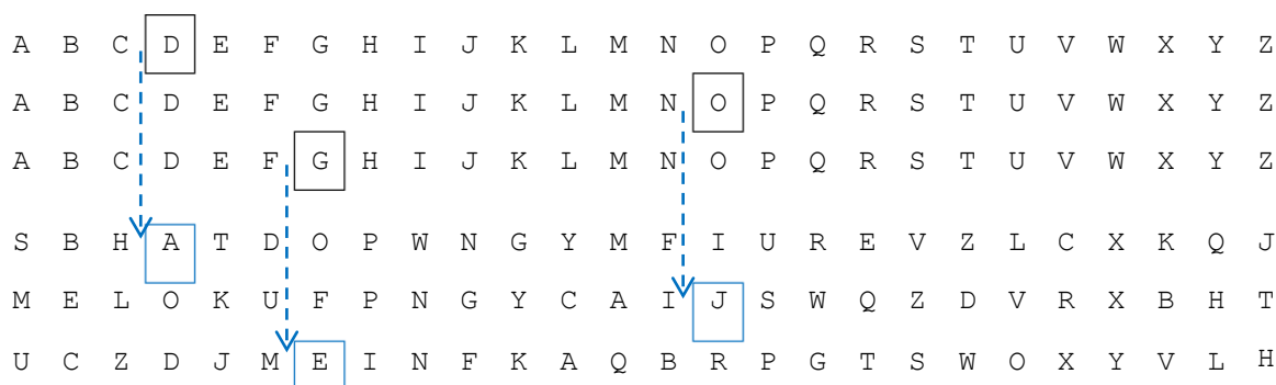
Рис. 1. Триграмний шифр
