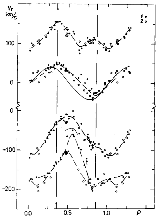
Рис. 6. Променеві швидкості профілю лінії H_\alpha у зміні з орбітальною фазою (1 – ПЗЗ-спостереження 1990-91 рр., 2 – 1985-89 рр.): графіки вгорі та внизу стосуються відповідно червоних та фіолетових піків емісії; другий графік зверху – центру емісії (суцільна крива відповідає орбітальному руху акретора); другий графік знизу – А-абсорбції. Стрілками та рисками відзначено фази 0.35P та 0.85P спостережень полюсів магнітного поля донора.
